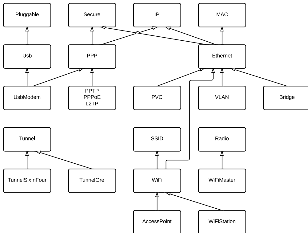
Рисунок 3.1. Иерархия интерфейсов
